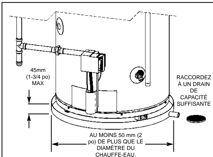
Figure 1 Installation-type du bac d'égouttement
