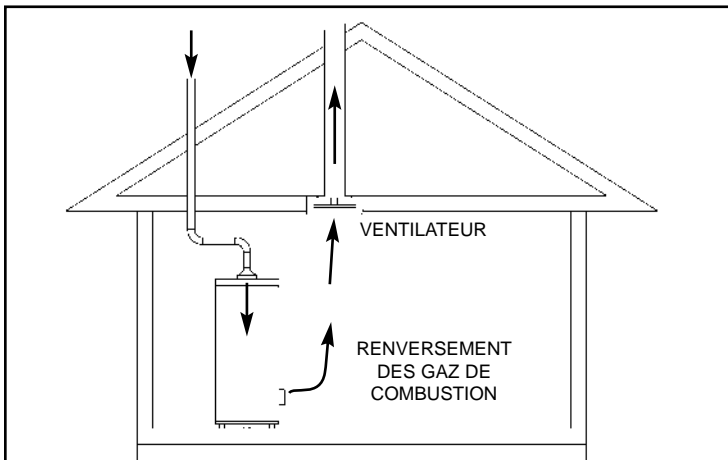
Figure 7 Appareil de ventilation
