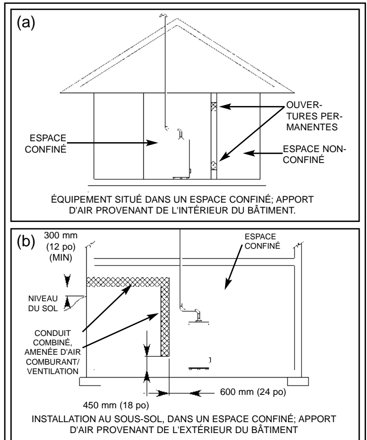
Figure 5 Conduits et ouvertures d'approvisionnement en air comburant (Canada)
