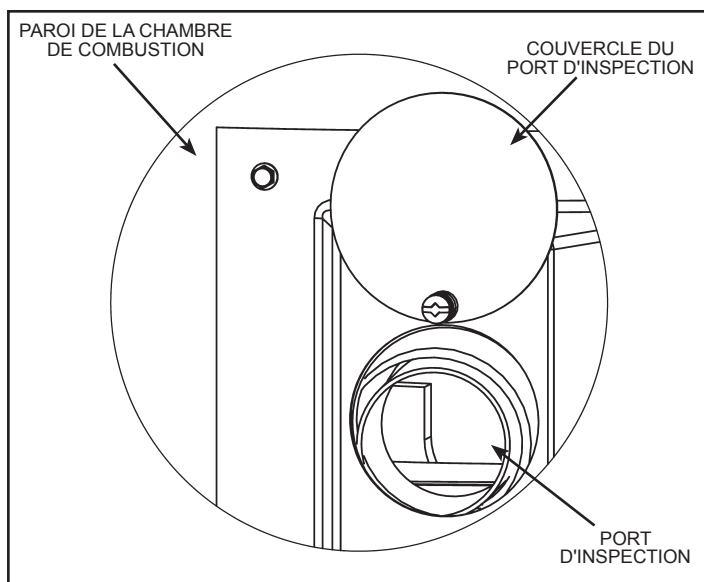
Figure 11. Port d'inspection (657, 717)
