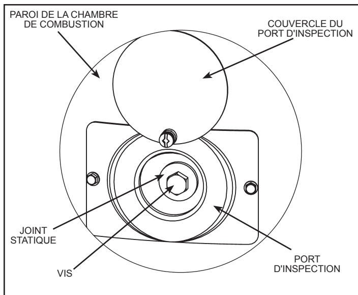
Figure 10. Port d'inspection (307, 307V, 507)
