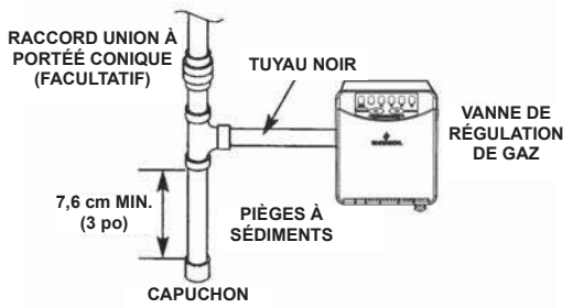
Figure 28. Tuyauterie de gaz avec tuyau en fer noir jusqu'à la commande de gaz
